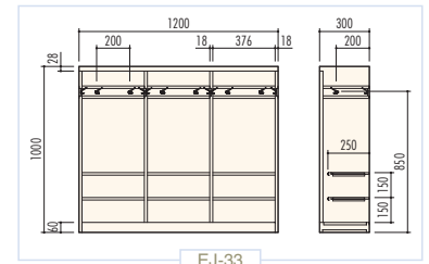
● EJ-33 / 園児用オープンロッカー(3列6人用) H1000×W1200×D300 (h912×w376) 1マス2人用、棚板[2]、フック[4]付
