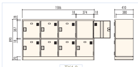
● TY4-2 / 生徒用ロッカー(4列2段8人用) H890×W1586×D410 (h387×w374) 横中仕切板差込構造、扉(補強付)、名札差プレス加工
