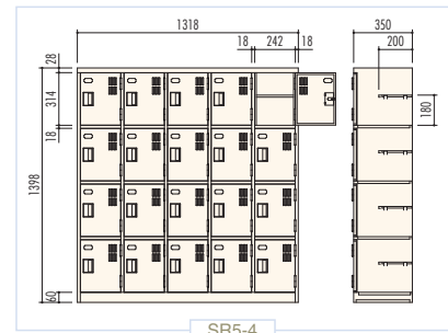
◆ SR5-4 / シューズケース(5列4段20人用) H1398×W1318×D350 (h314×w242) 横中仕切板差込構造、名札差プレス加工、中棚付
